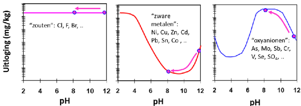
Figuur 4.1 uitloggedrag voor verschillende groepen stoffen en het effect als de pH verandert van ongeveer pH 12 naar pH 8 (weergegeven met een pijl) (overgenomen uit Dijkstra, (2024)).
