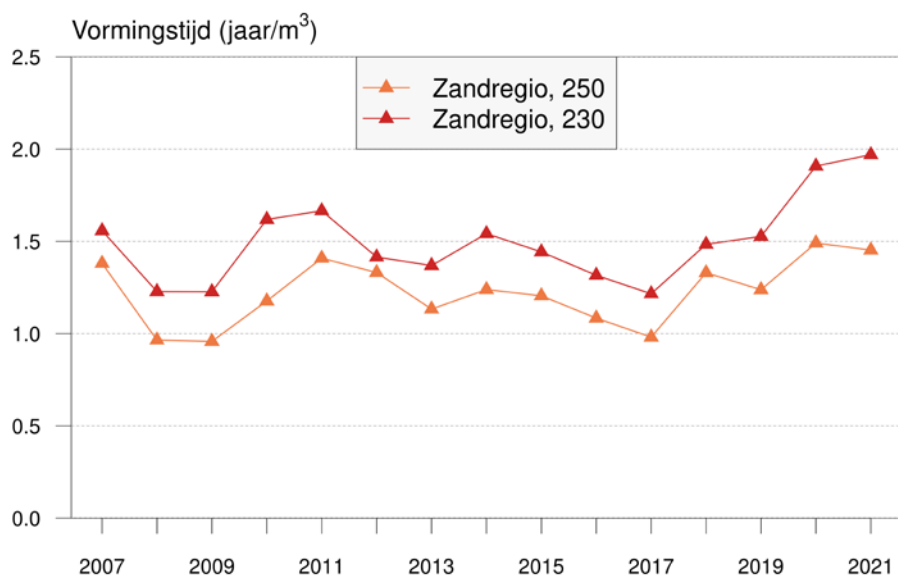
Figuur 4.18 Vormingstijd van de bovenste meter van het grondwater (jaar/m³) op bedrijven in het derogatiemetnet in Zand 250 en Zand 230.
