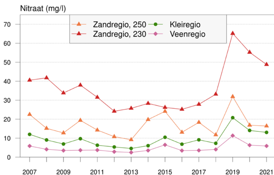
Figuur 4.15 Gemiddelde nitraatconcentratie (mg/l) in slootwater op bedrijven in het derogatiemetnet in de drie regio's in de periode 2007-2021.
