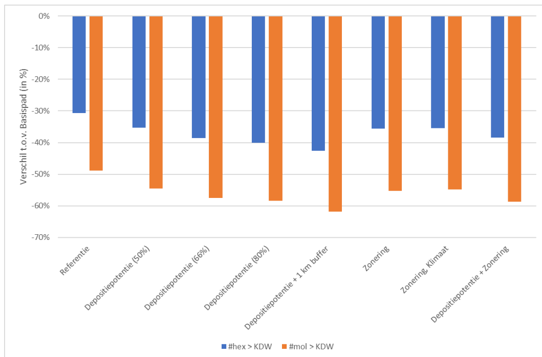
Figuur 18 Percentuele verschillen in het effect van emissiereducties volgens verschillende varianten ten opzichte van het Basispad, voor het aantal hexagonen boven de KDW en de hoeveelheid stikstof in mol boven de KDW in Nederland.
