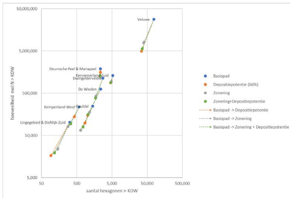
Figuur 19 Effect van emissiereducties volgens verschillende varianten, uitgedrukt in het aantal hexagonen boven de KDW (x-as) en de hoeveelheid stikstof in mol boven de KDW (y-as) voor enkele gebieden in Nederland (n.b. x- en y-as zijn logaritmisch).
