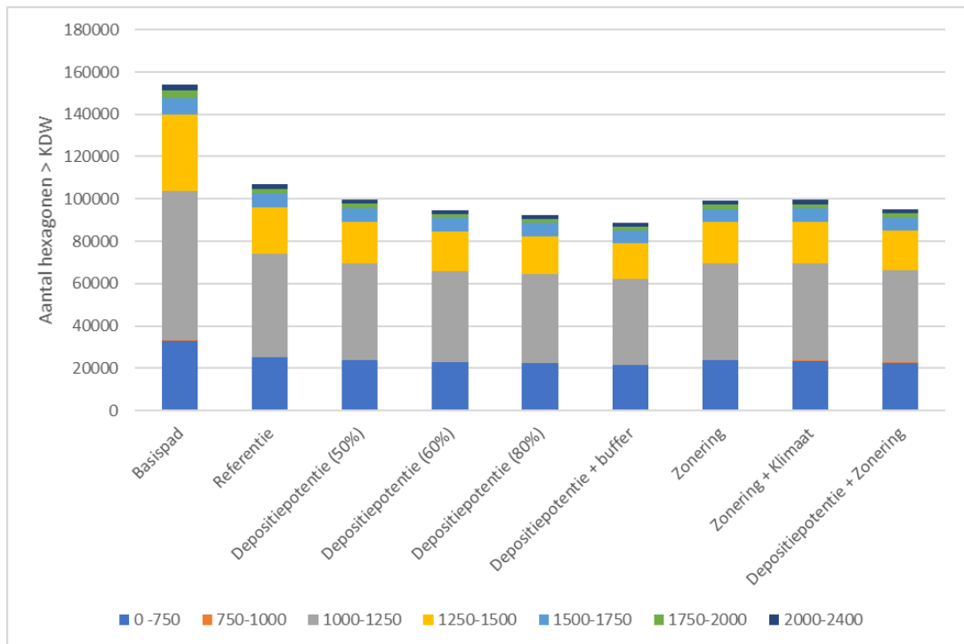
Figuur 16 Aantal hexagonalen boven de KDW voor verschillende KDW-klassen en voor de verschillende varianten.
