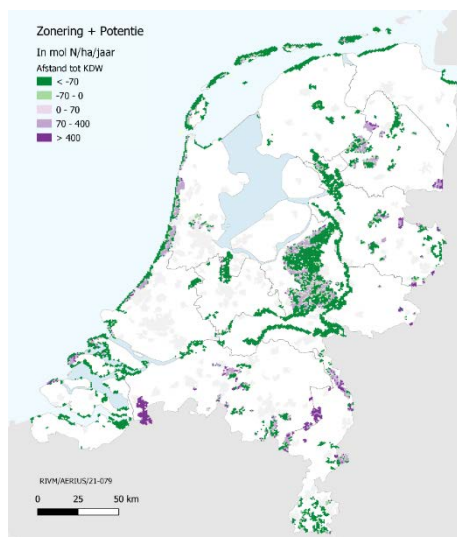
Figuur 14 Ruimtelijk beeld van de afstand tot de KDW volgens de Depositiepotentie + Zonerings variant.
