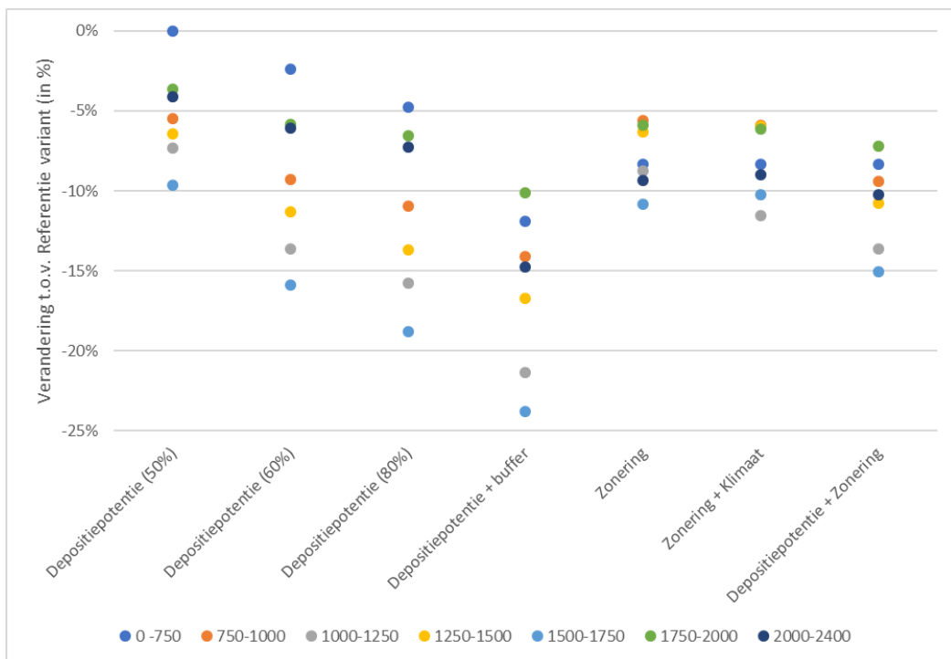
Figuur 17 Verandering (in %) van het aantal hexagonalen boven de KDW voor verschillende KDW klassen ten opzichte van de Referentie variant.
