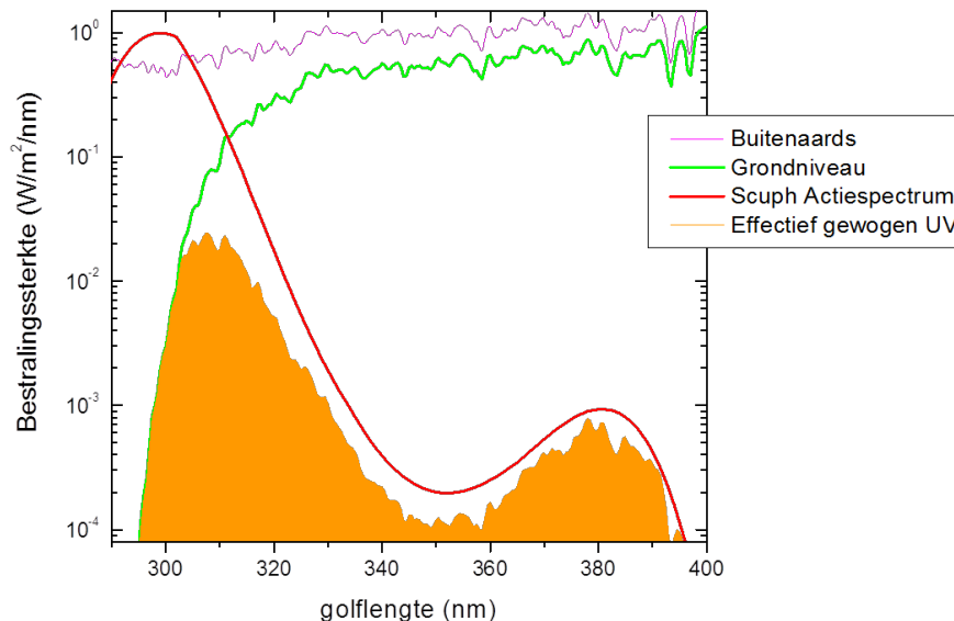
Figuur 7.1 Vergelijking van het buitenaards zonnenspectrum met een meting van het zonnenspectrum op grondniveau (groene curve), en de biologische effectiviteit van UV-straling, hier geïllustreerd voor de inductie van huidkanker (de rode curve). In de fotobiologie wordt die curve aangeduid als actiespectrum (hier getoond: actiespectrum SCUP-h voor huidkanker (de Gruijl en van der Leun, 1994)). Vermenigvuldiging van het actiespectrum met het spectrum op grondniveau en sommatie over alle UV-golflengten geeft de voor huidkanker relevante bestralingssterkte: het oranje oppervlak in de figuur. Merk op dat de Y-as logaritmisch is, en dat de bestralingssterkte op grondniveau van 315 nm naar 295 nm meer dan een factor 1000 vermindert.
