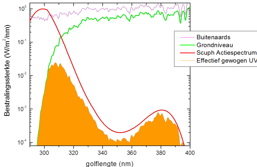
Figuur 5.1 Vergelijking van het buitenaards zonnenspectrum met een meting van het zonnenspectrum op grondniveau (groene curve; meting RIVM), en de biologische effectiviteit van UV-straling, hier geïllustreerd voor de inductie van huidkanker (de rode curve). In de fotobiologie wordt die curve aangeduid als actiespectrum (hier getoond: actiespectrum SCUP-h voor huidkanker (de Gruijl en van der Leun, 1994)). Vermenigvuldiging van het actiespectrum met het spectrum op grondniveau en sommatie over alle UV-golflengten geeft de voor huidkanker relevante bestralingssterkte: het oranje oppervlak in de figuur. Merk op dat de Y-as logaritmisch is, en dat de spectrale bestralingssterkte op grondniveau van 315 nm naar 295 nm meer dan een factor 1000 vermindert.
